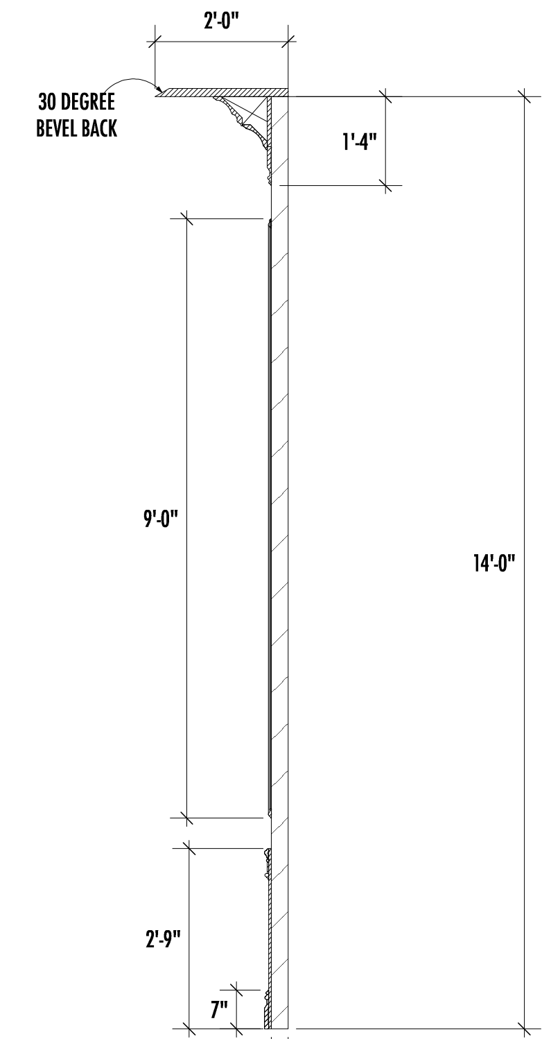
CL SECTION-WALL A Scale: 1/2" = 1'-0"
